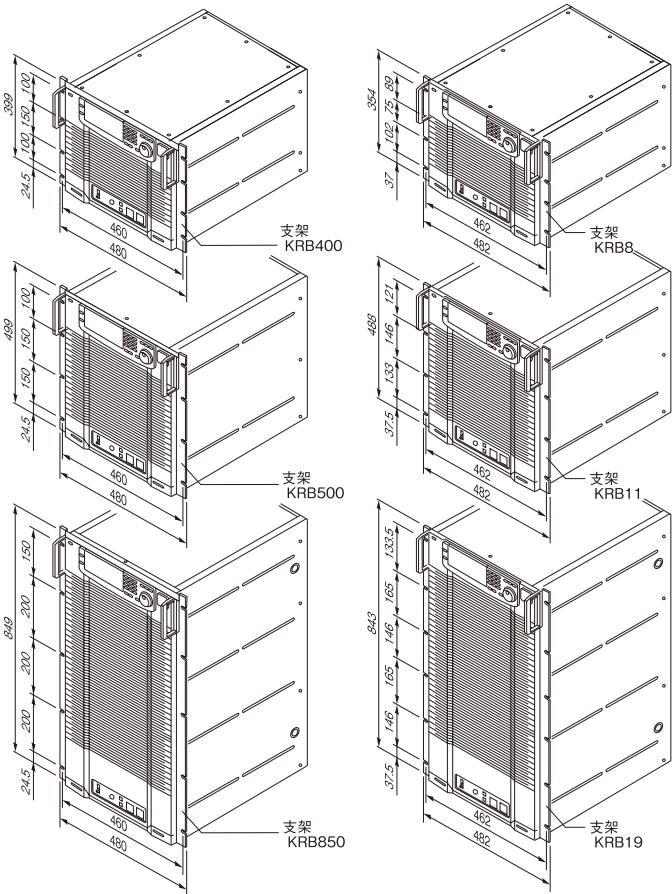
单相 & 三相类型 (例: PCR6000W²)
